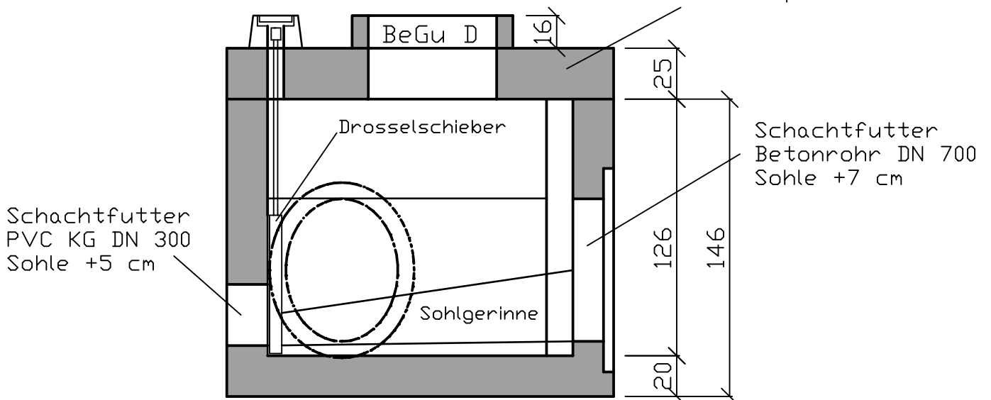
Schnitt A-A
